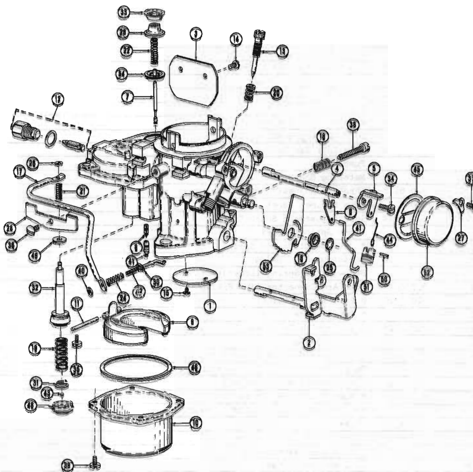
CARBURETOR 64-65 01 (LHE)
